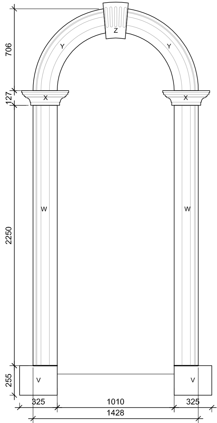
1010 ARCH ELEVATION Scale: 1:20
